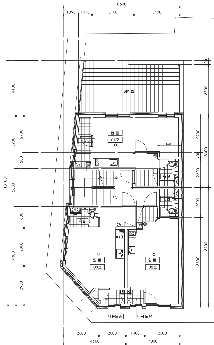
4층 평면도
