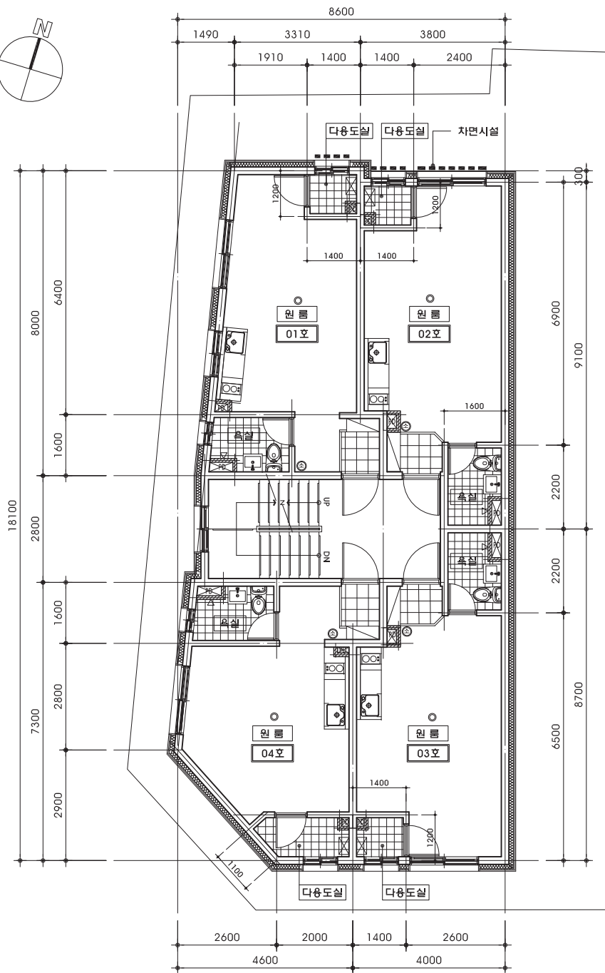
2층,3층 평면도
